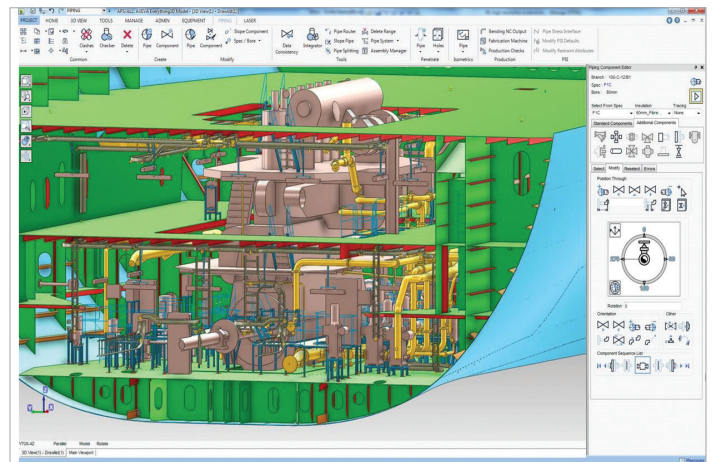
三维视图中的船体数据
