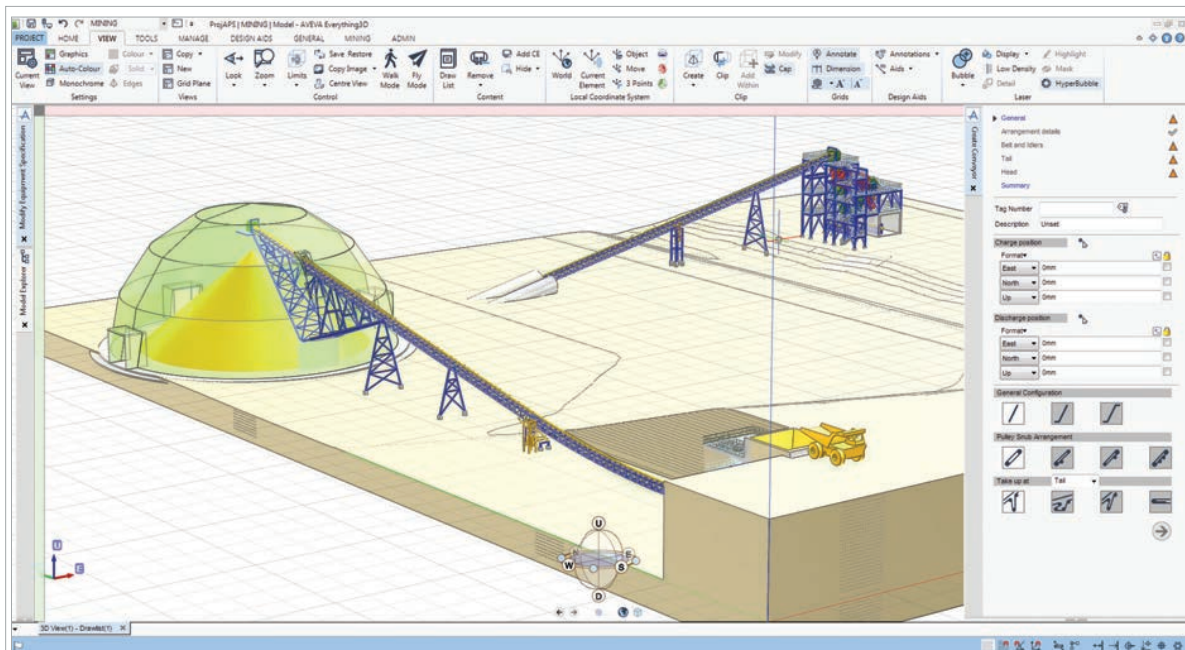
AVEVA E3D Design具有友好的综合界面,包含煤炭运输机布局设计
