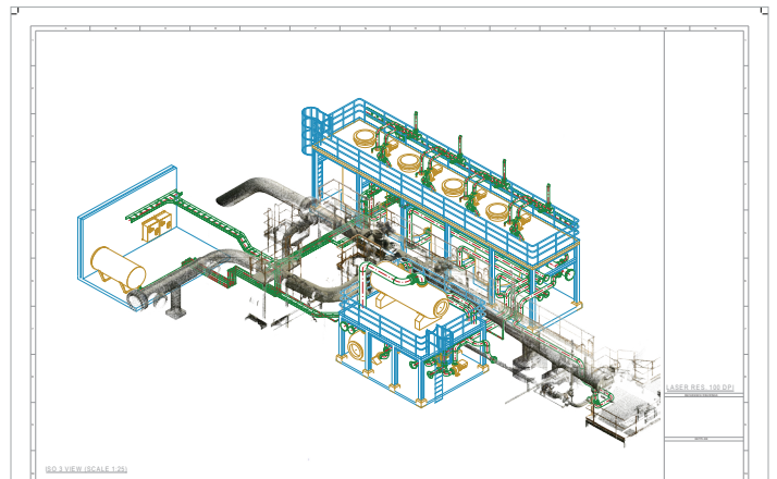
DRAW中的激光数据避免了对现有结构的改造
