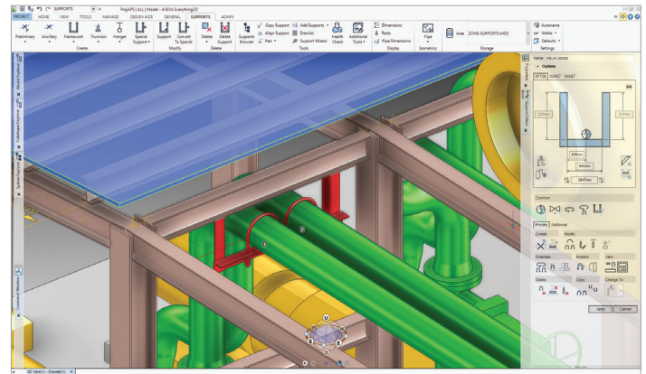
可以把详细的信息快速添加到设计中
