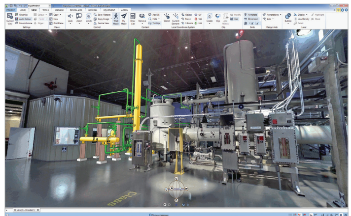
集成到三维视图的激光扫描数据
