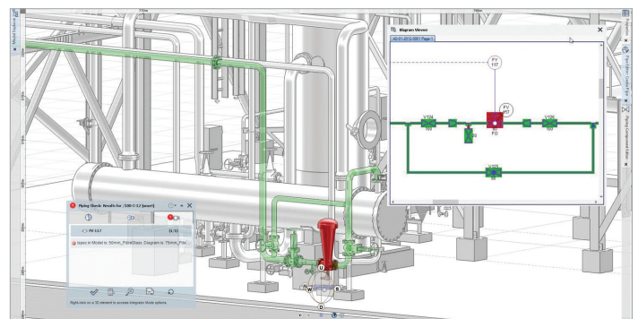
一体化工程——比较和更新P&ID和三维模型
