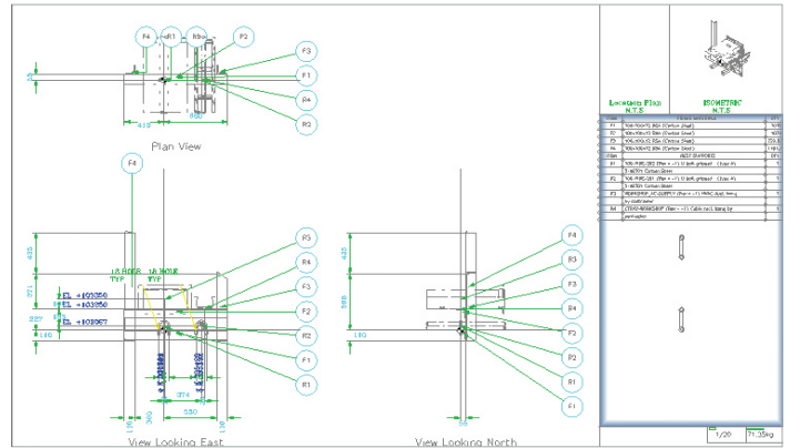
自动生成的管道支撑图
