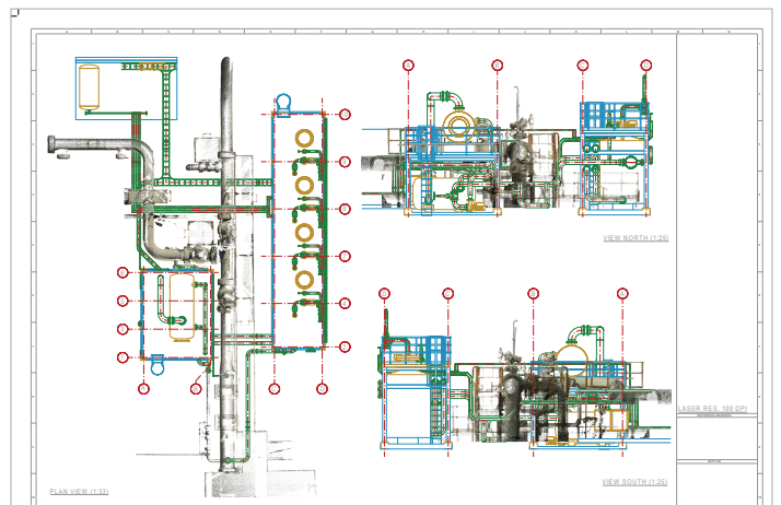
布局图和规划图可包含激光数据
