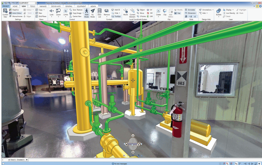
AVEVA E3D让设计人员在一个激光扫描数据与新的三维设计融合在一起的环境中工作
