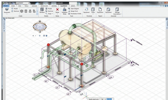
三维视图中可以包含网格线、尺寸和注释
